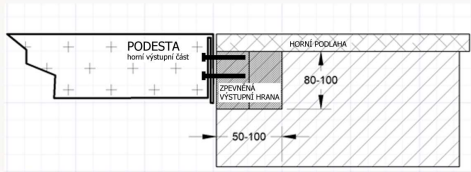
Detail kotvení podesty (pohled z boku)
