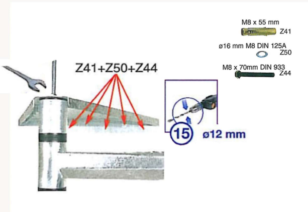
Detail kotvení podesty (pohled z boku)
